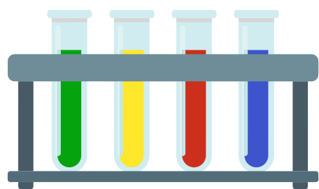
Sodiopropynol
