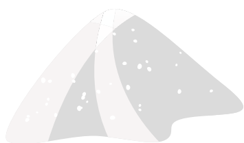
Magnesiumsulfat
